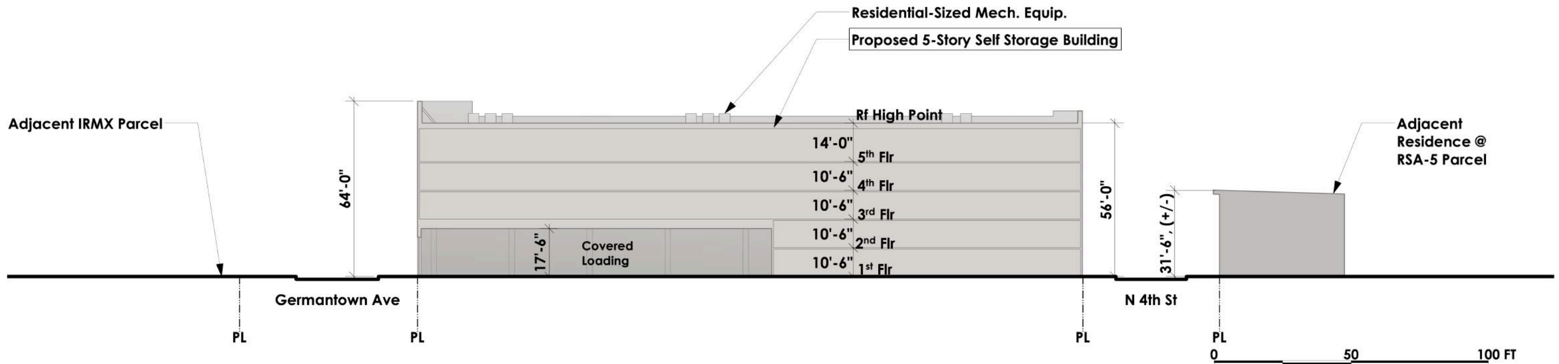
Section A - Longitudinal Section
